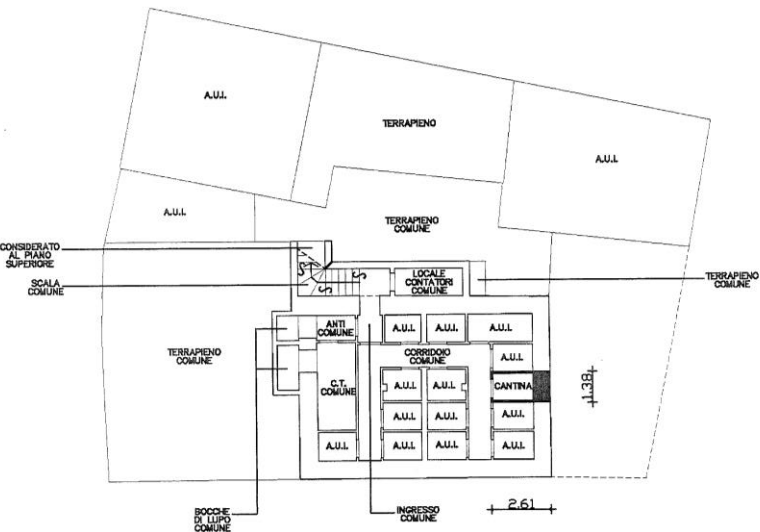
PIANTA PIANO INTERRATO H = 2,20 mt
